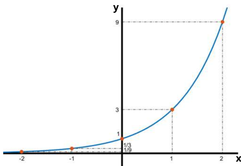
Gráfico 2: f(x) = 3^x
