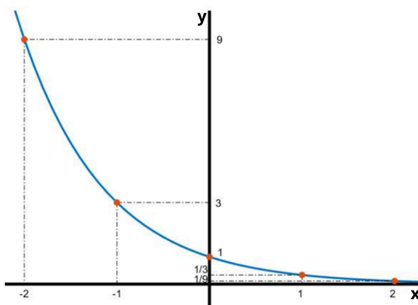
Gráfico 4: f(x) = \left(\frac{1}{3}\right)^x
