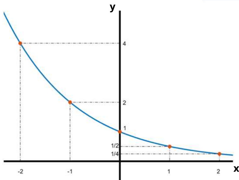
Gráfico 3: f(x) = \left(\frac{1}{2}\right)^x
