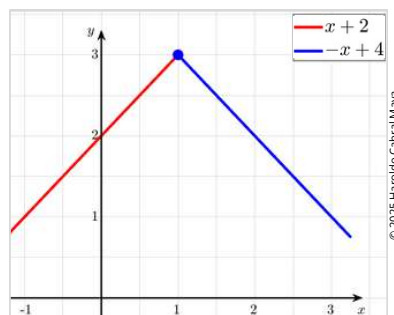
Figura 1: Gráfico da função definida por partes composta por duas semirretas, uma crescente e outra decrescente.
