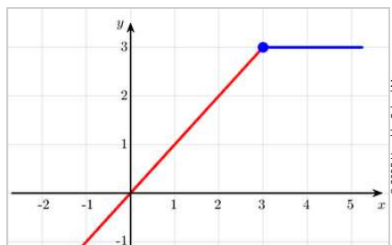
Figura 3: Gráfico de uma função definida por partes.
